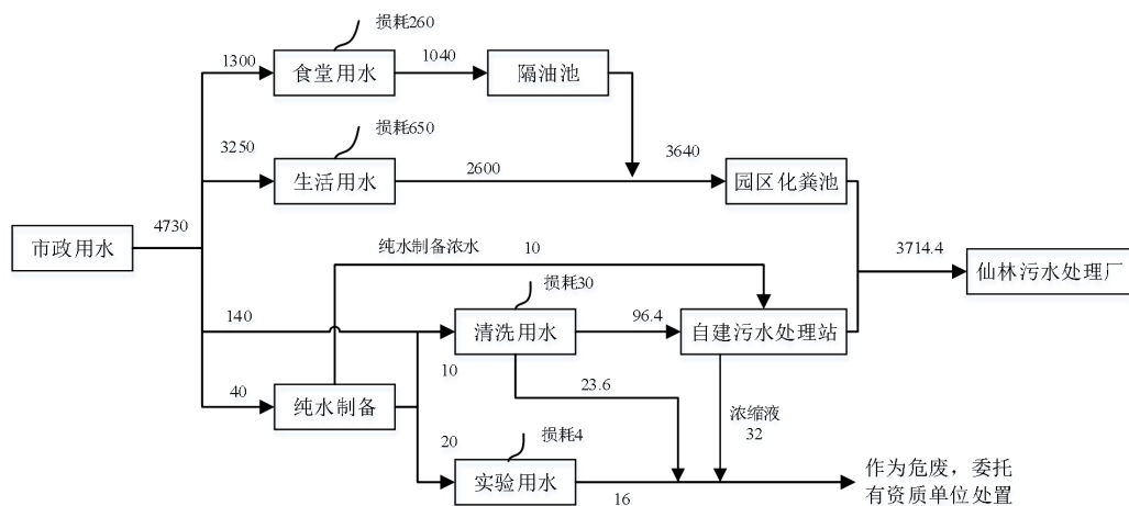
图2-1 全厂水量平衡图 (t/a)
