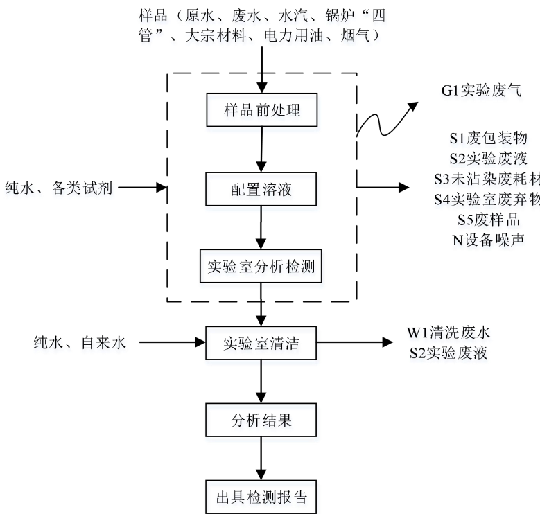
图2-2 检测工艺流程及产污环节图
